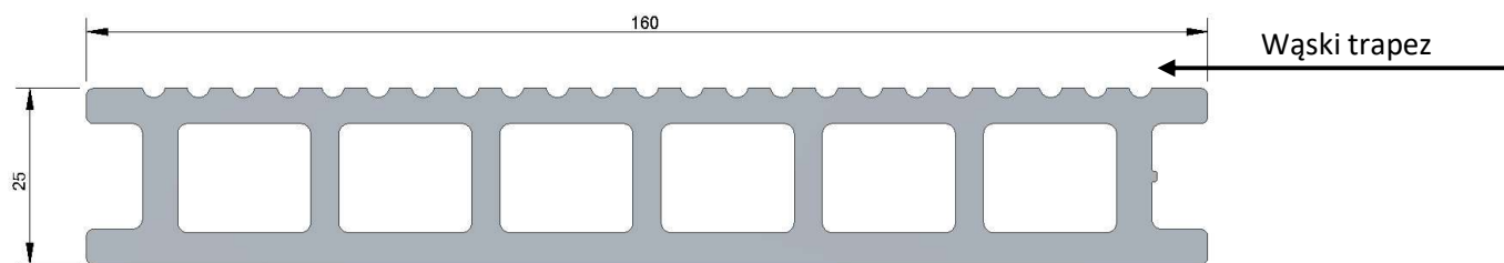
Rys 1. Przekrój poprzeczny deski EVO PRO
